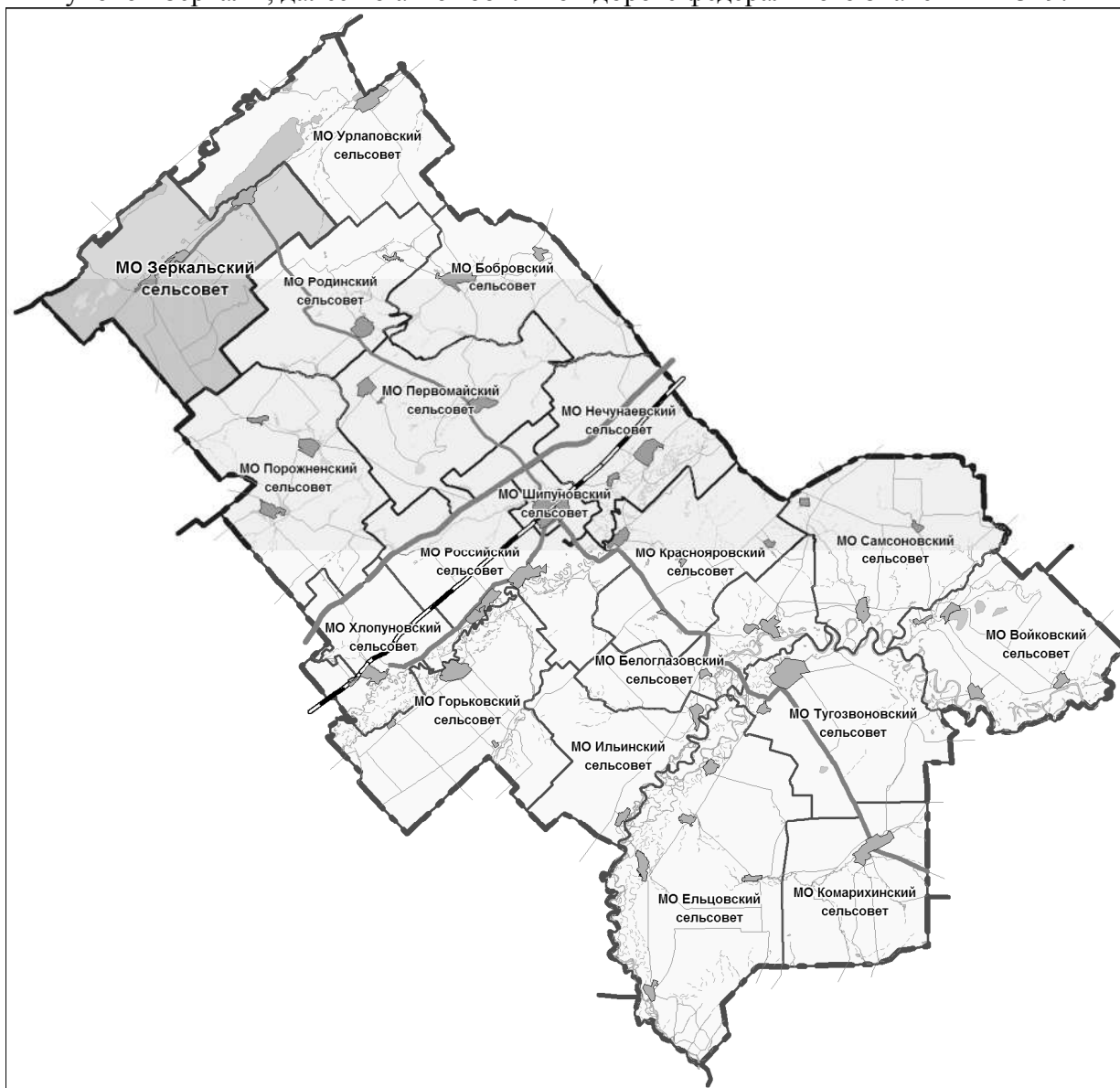
Рисунок 1. – Схема расположения муниципального образования Зеркальский сельсовет на территории Шипуновского района
